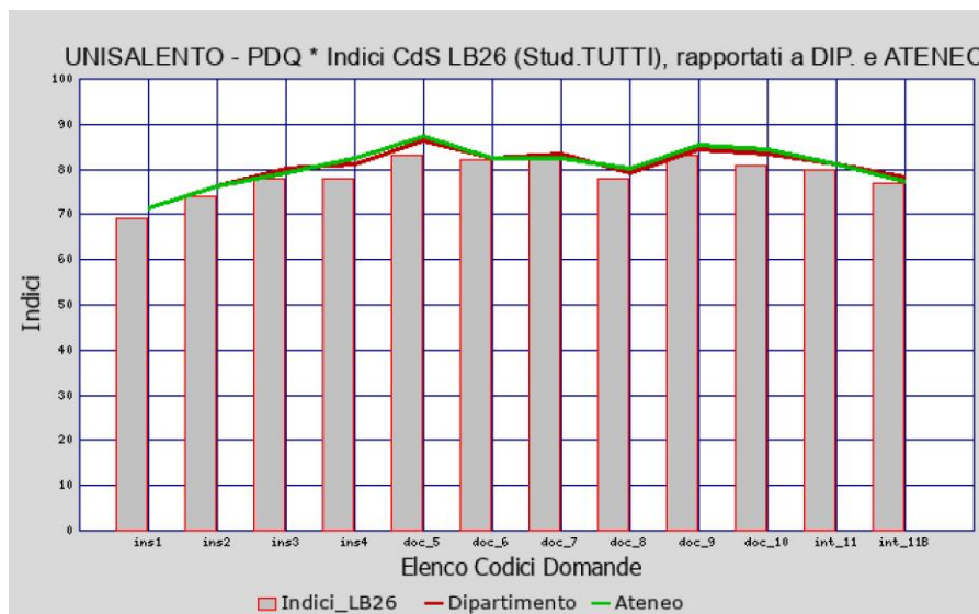
Fig. 1. Indici CdS LB26/2016, tutti gli STUDENTI, rapportati a DIPARTIMENTO e ATENEO
